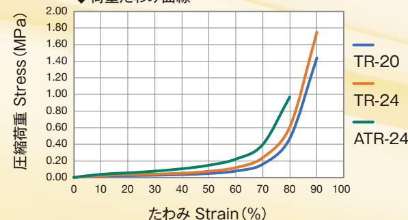
◆荷重たわみ曲線
